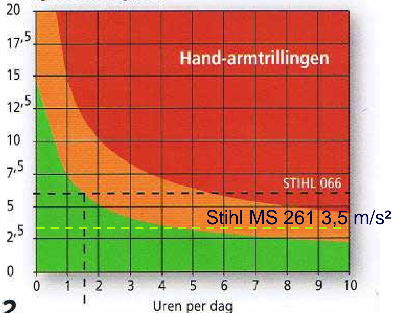
Trillingsblootstelling (m/s 2 )
